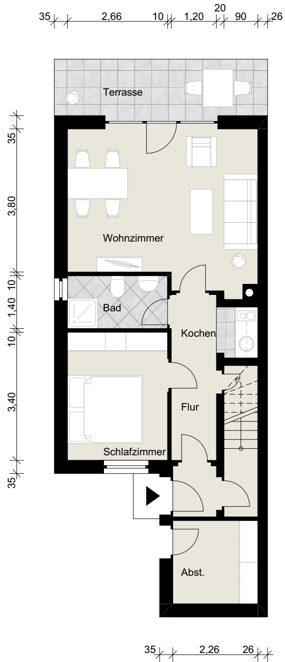
Grundriss EG
